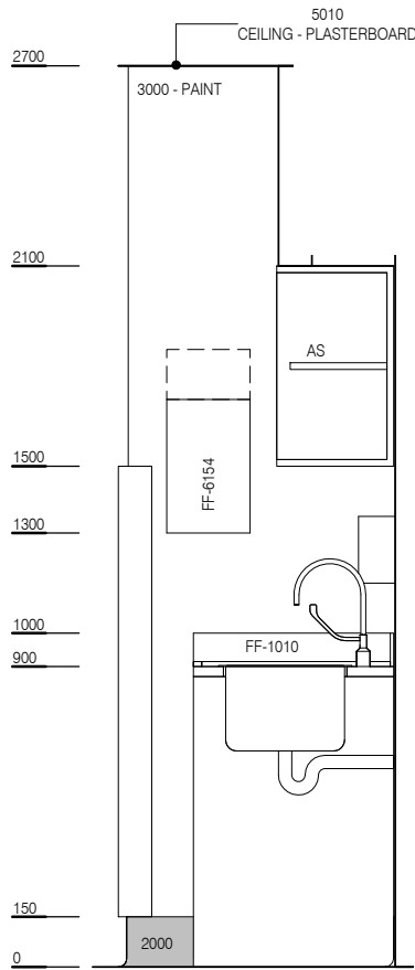
ELEVATION 1
