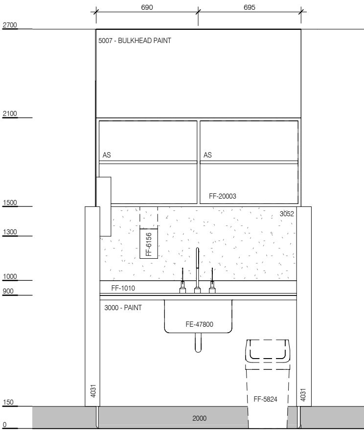
ELEVATION 2
