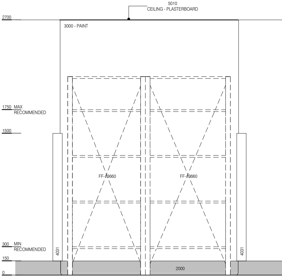
ELEVATION 2
