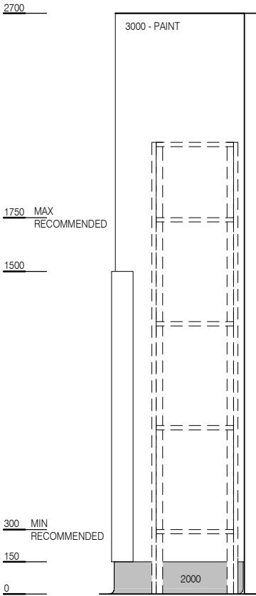
ELEVATION 1
