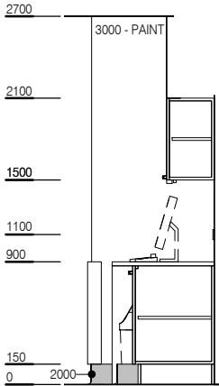
ELEVATION 1
