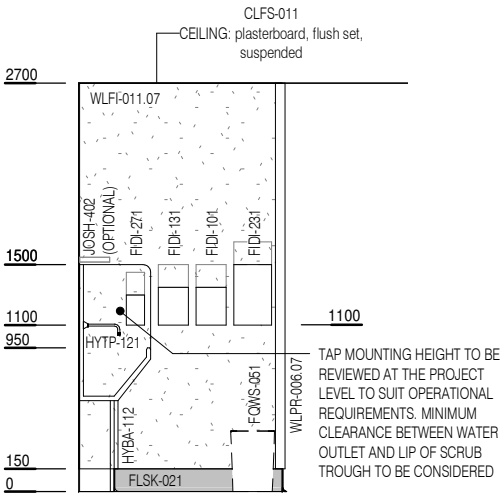
ELEVATION 2
