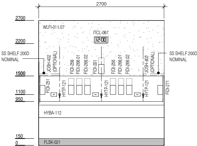
ELEVATION 1
