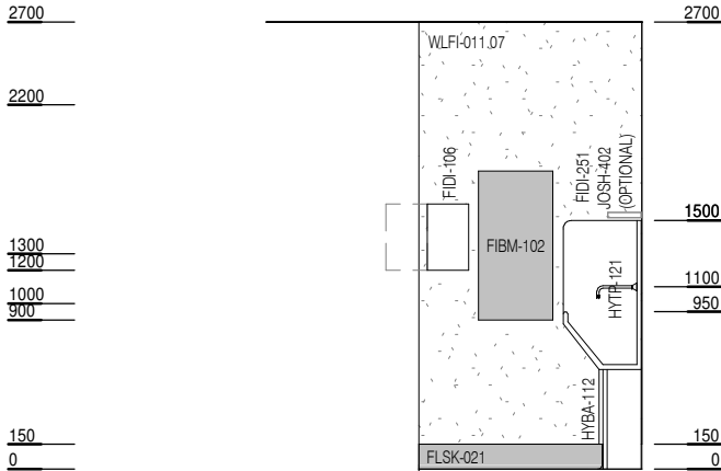
ELEVATION 3
