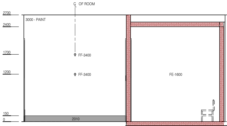
ELEVATION 4
