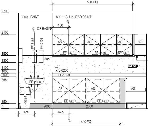
ELEVATION 4
