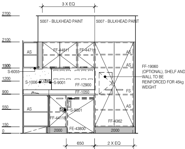
ELEVATION 1
