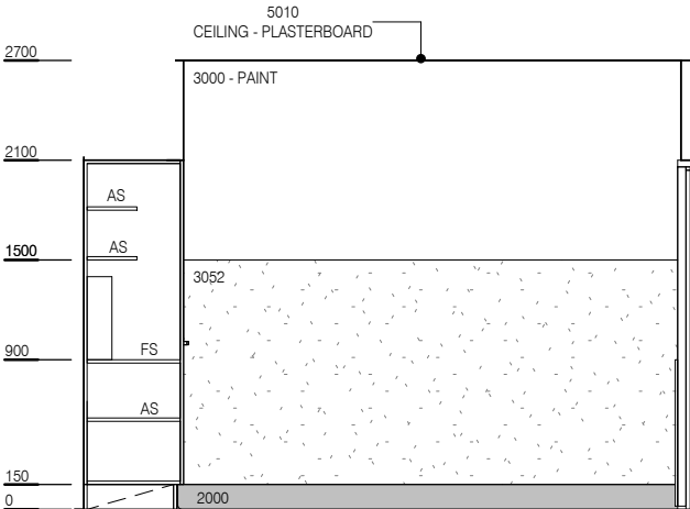
ELEVATION 2
