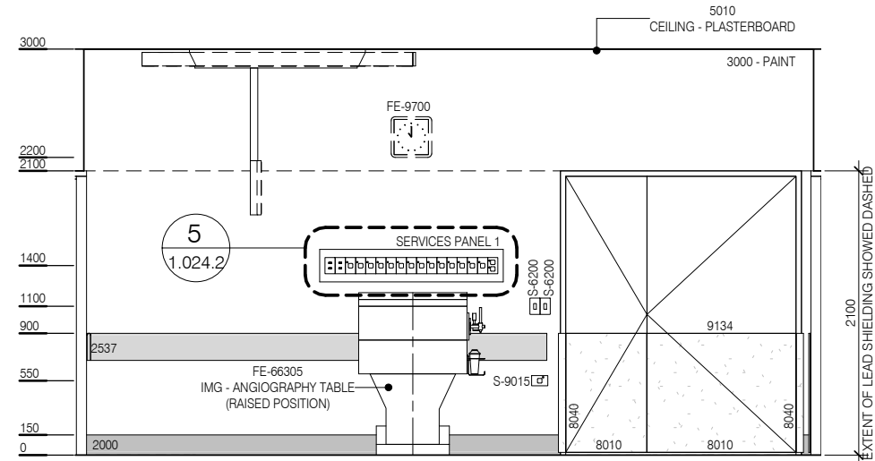
ELEVATION 3
