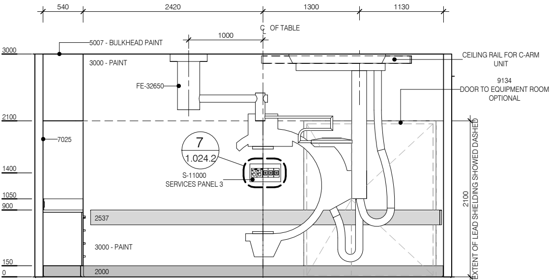
ELEVATION 1
