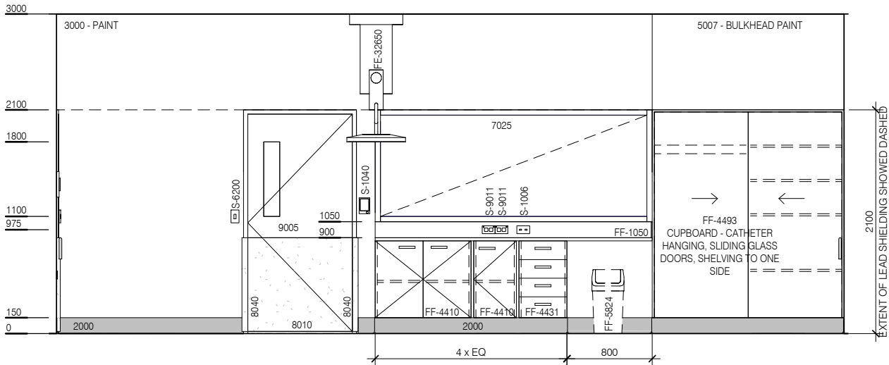
ELEVATION 4
