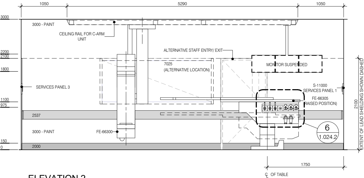
ELEVATION 2
