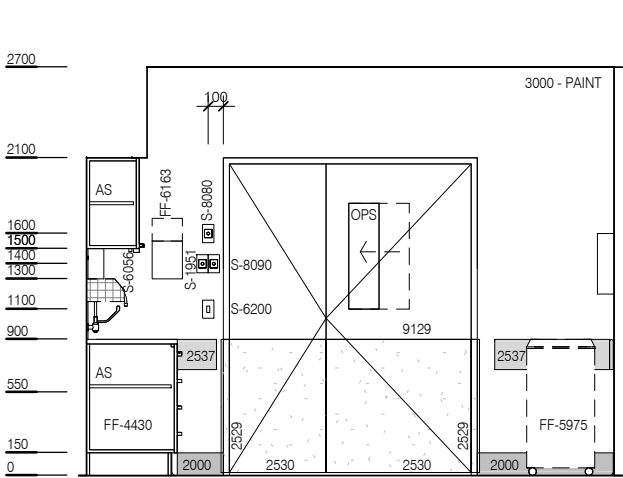
ELEVATION 3
