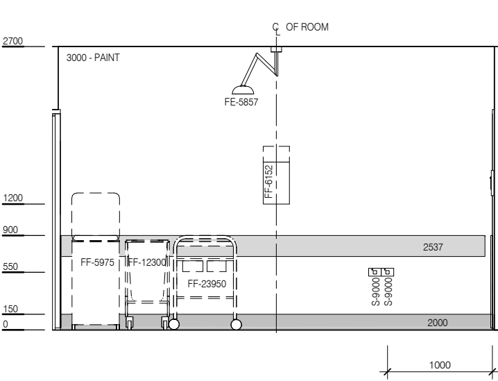
ELEVATION 4
