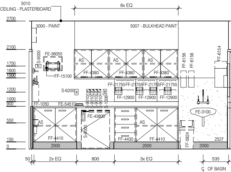
ELEVATION 2
