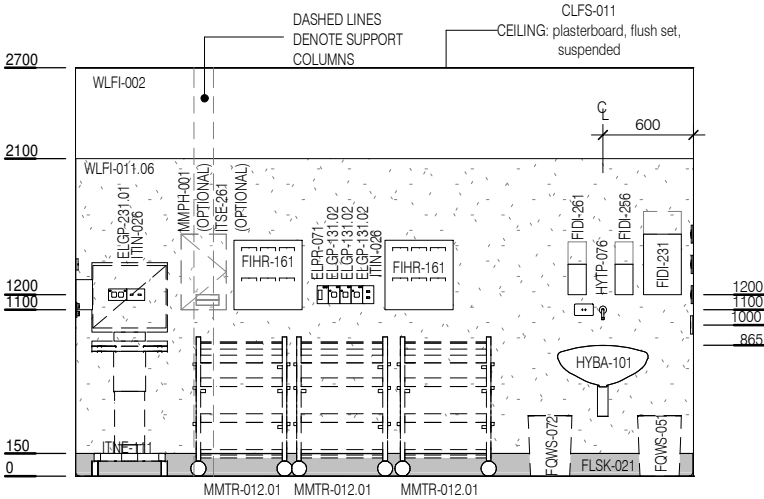
ELEVATION 2
