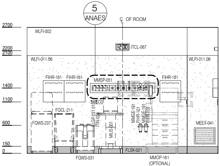
ELEVATION 4
