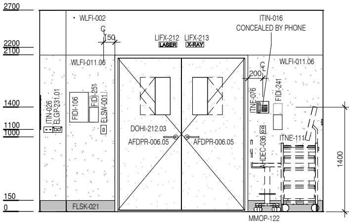
ELEVATION 1
