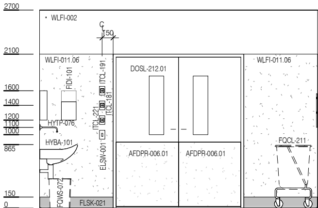
ELEVATION 3
