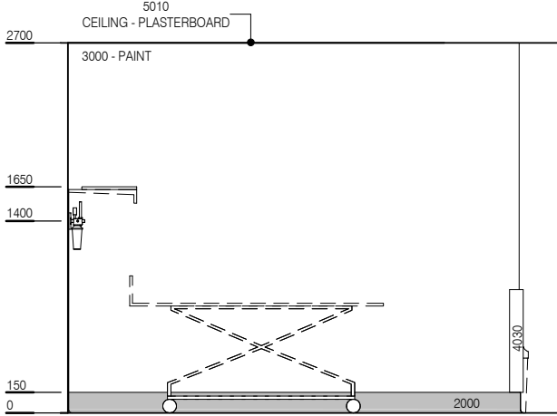
ELEVATION 2
