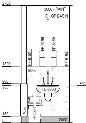
ELEVATION 5
