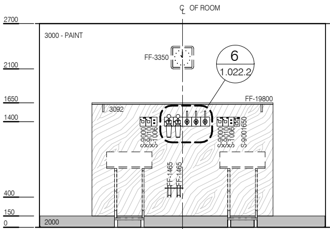
ELEVATION 1
