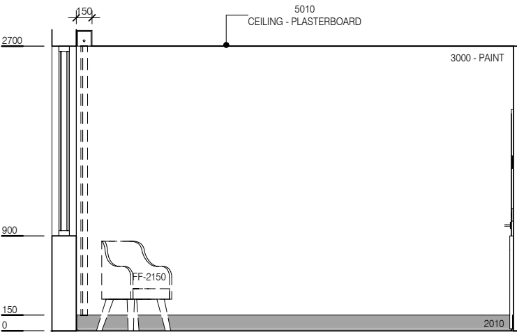
ELEVATION 2
