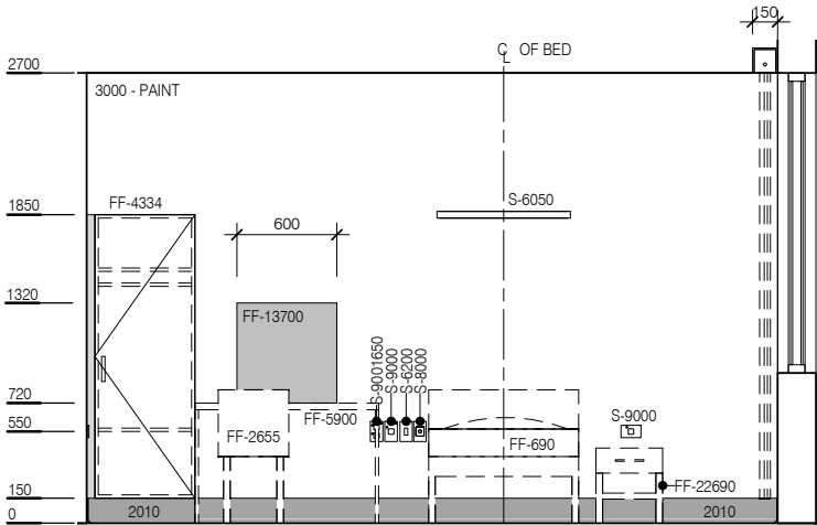
ELEVATION 4
