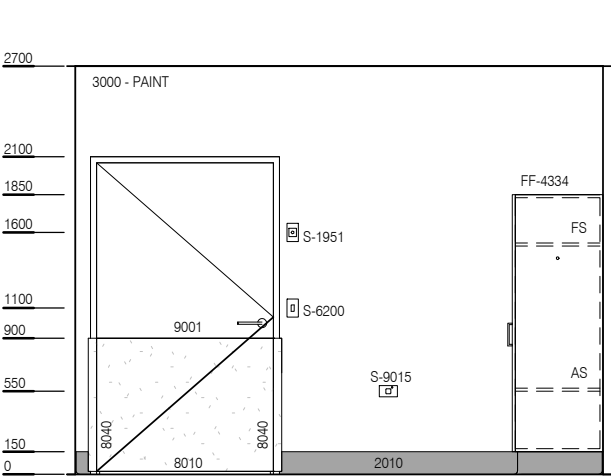
ELEVATION 3
