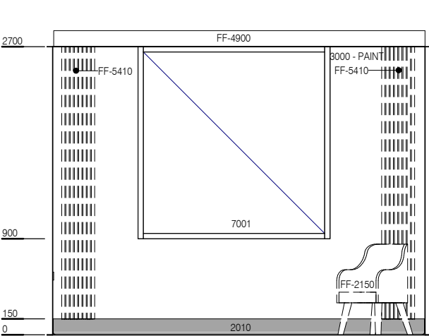
ELEVATION 1
