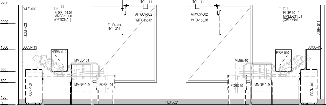
ELEVATION 1
