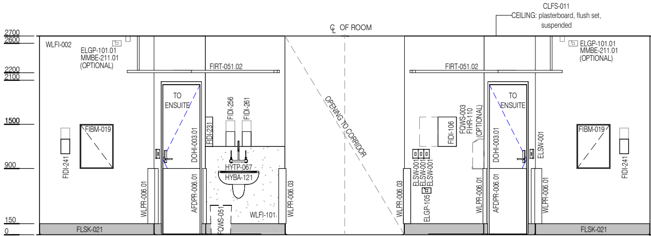
ELEVATION 3
