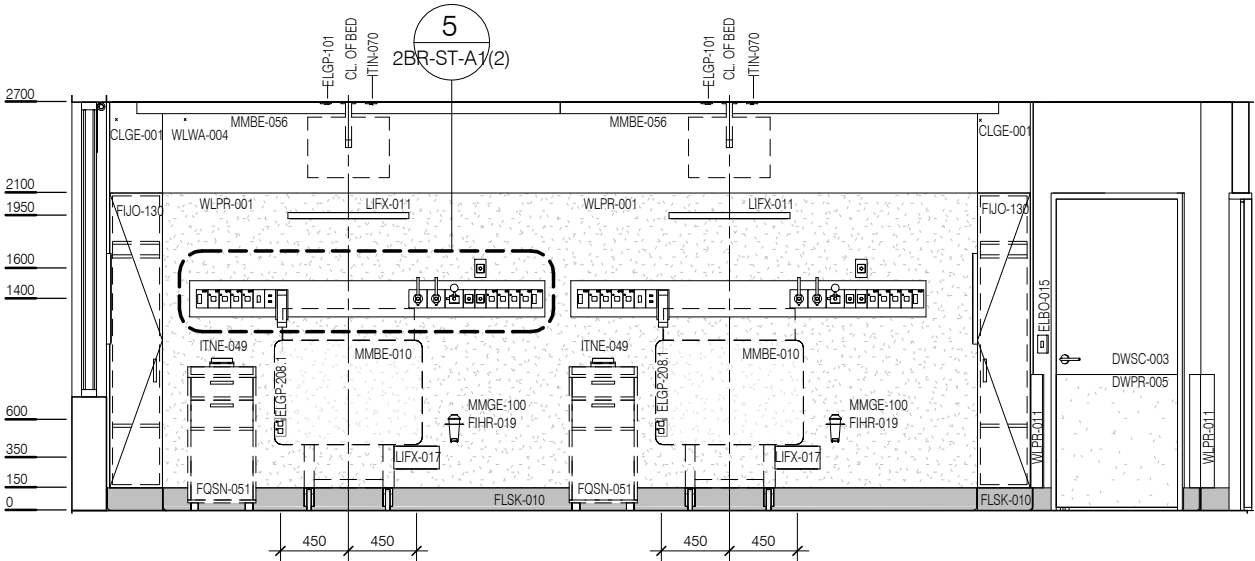
ELEVATION 2
