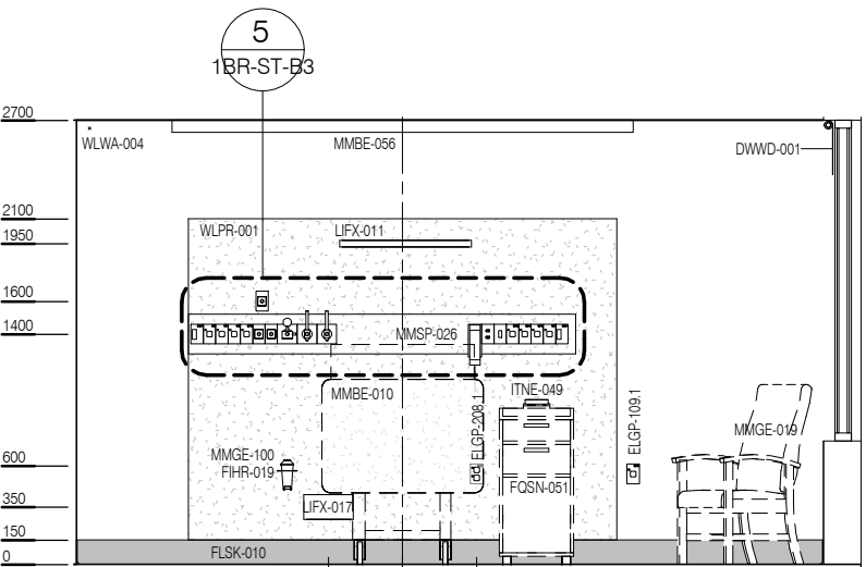
ELEVATION 4
