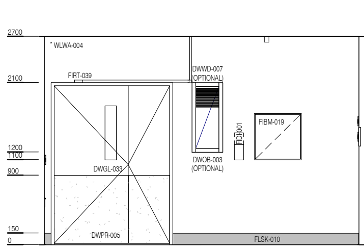
ELEVATION 3
