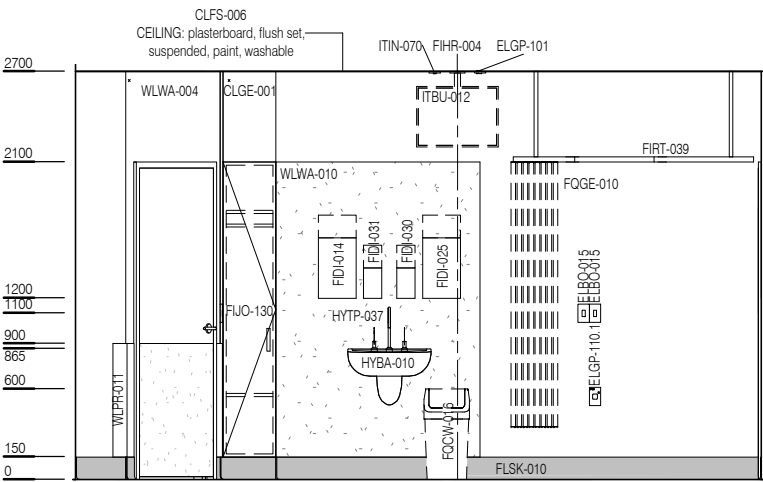
ELEVATION 2
