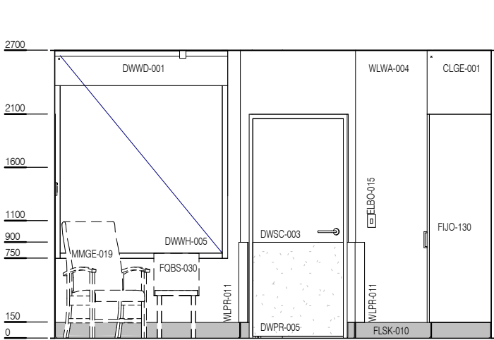
ELEVATION 1
