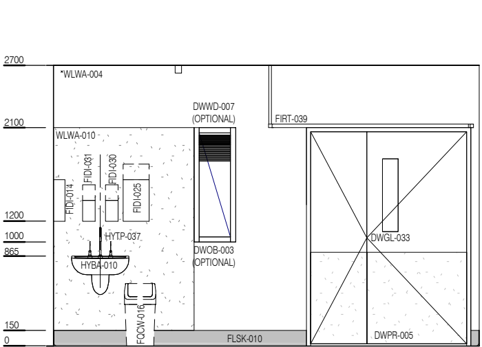
ELEVATION 3
