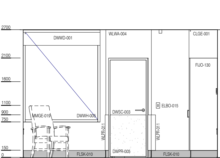
ELEVATION 1
