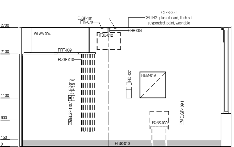
ELEVATION 4
