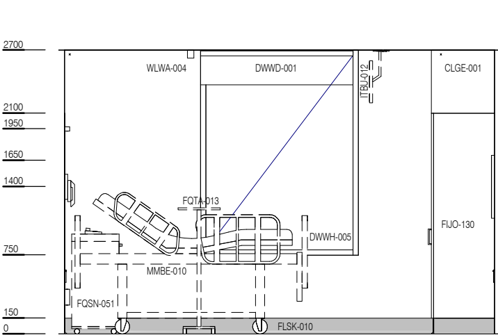
ELEVATION 1
