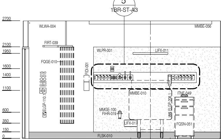
ELEVATION 4
