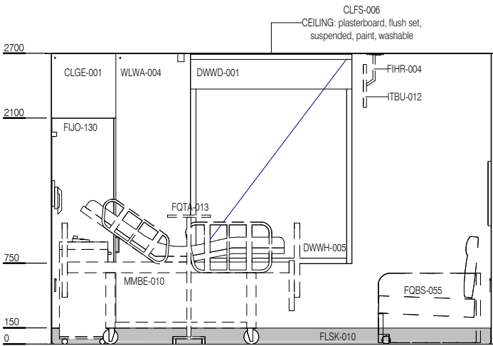
ELEVATION 1
