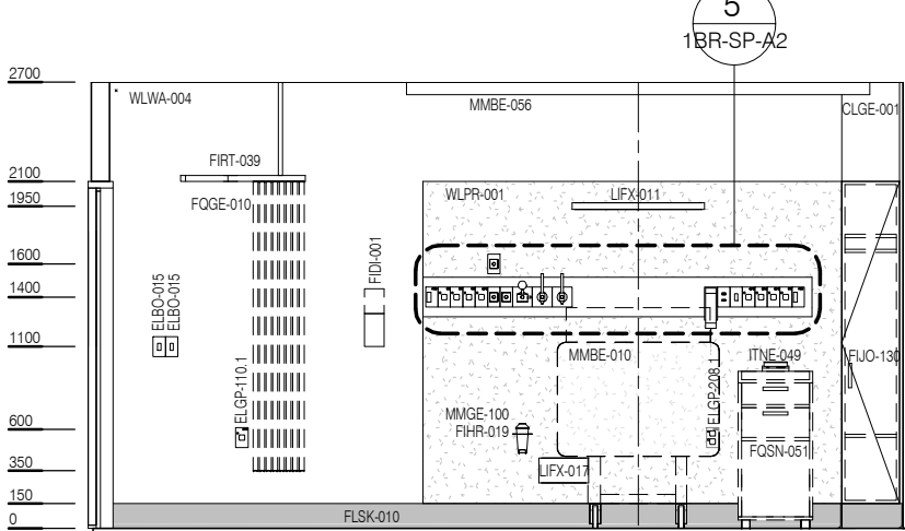
ELEVATION 4
