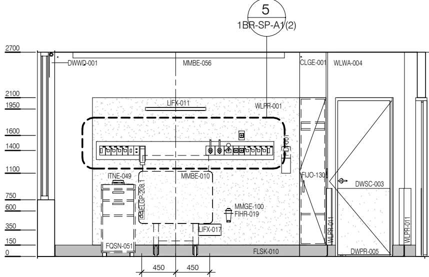
ELEVATION 2
