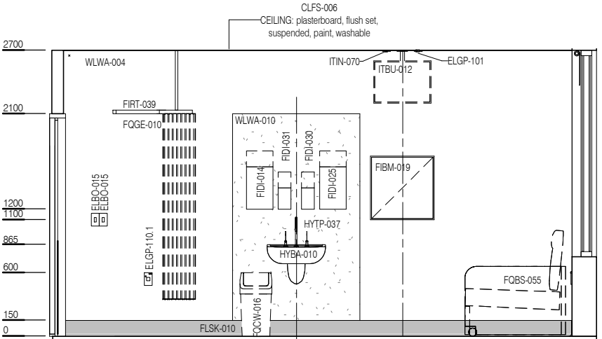
ELEVATION 4
