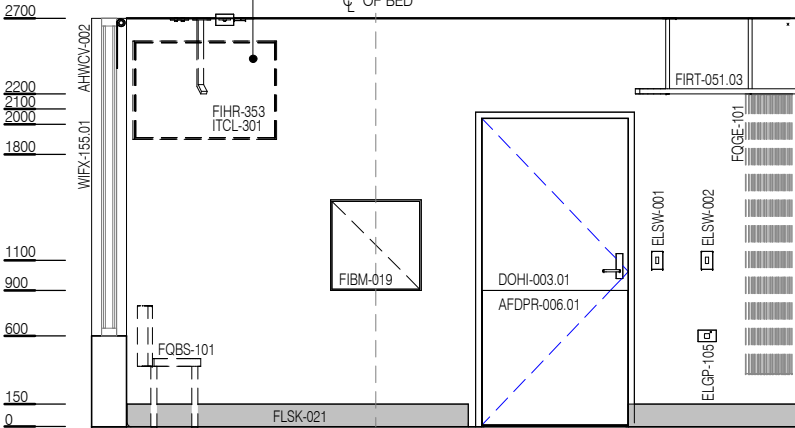
ELEVATION 2
