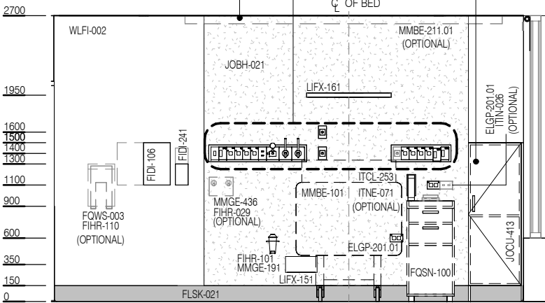
ELEVATION 4
