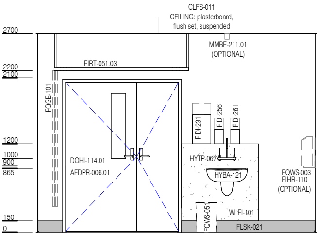
ELEVATION 3
