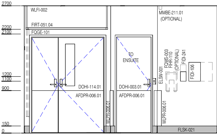
ELEVATION 3
