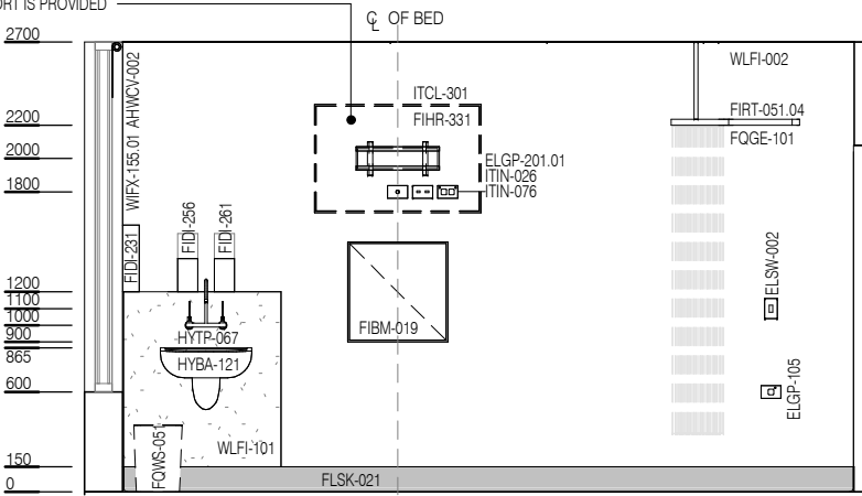
ELEVATION 2
