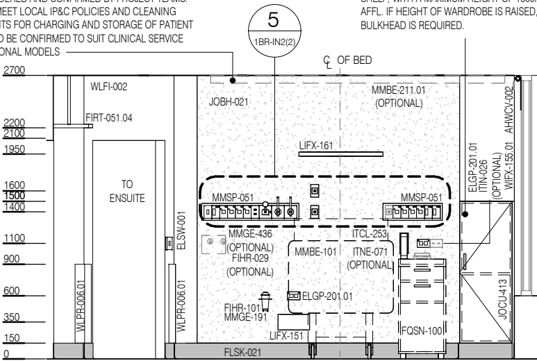
ELEVATION 4
