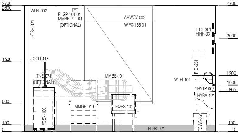
ELEVATION 1
