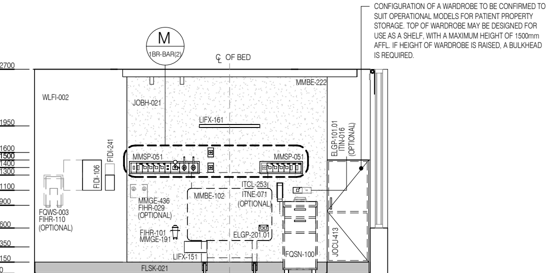
ELEVATION 4
