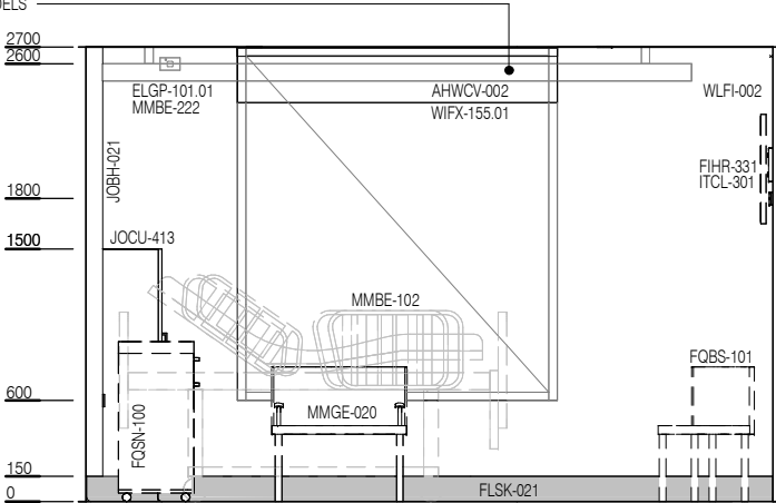
ELEVATION 1
