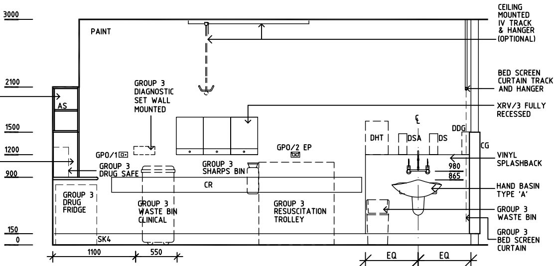
ELEVATION 2
