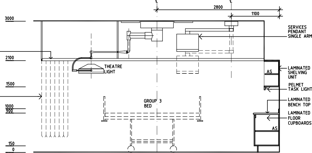
ELEVATION 2
