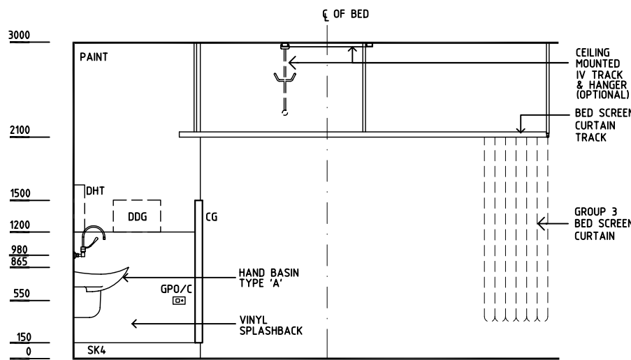
ELEVATION 1
