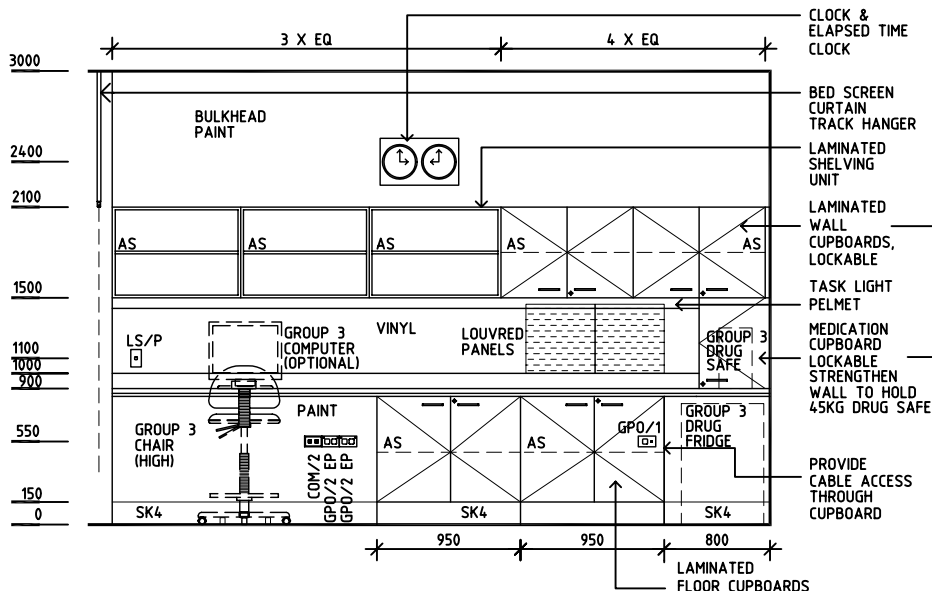
ELEVATION 1
