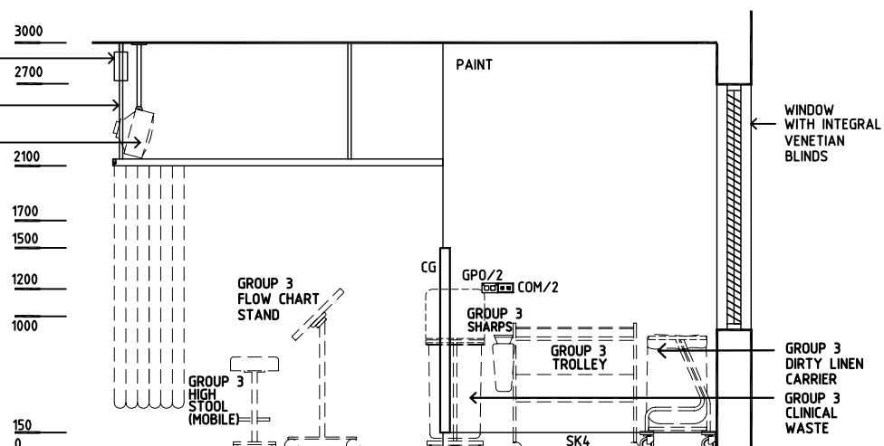
ELEVATION 4
