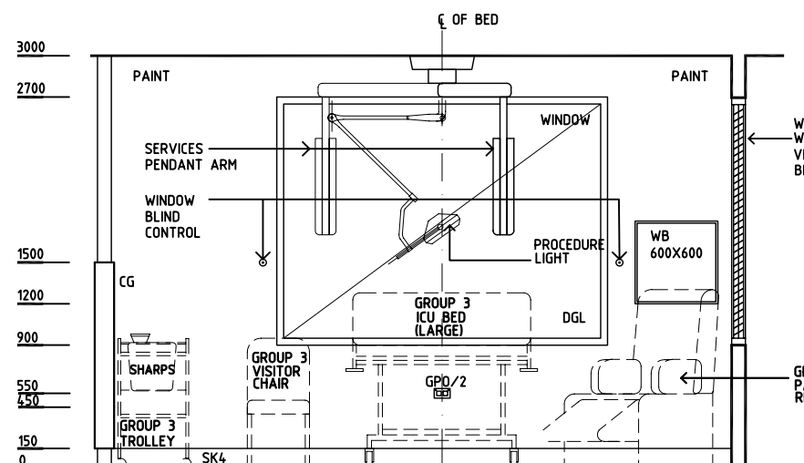
ELEVATION 1
