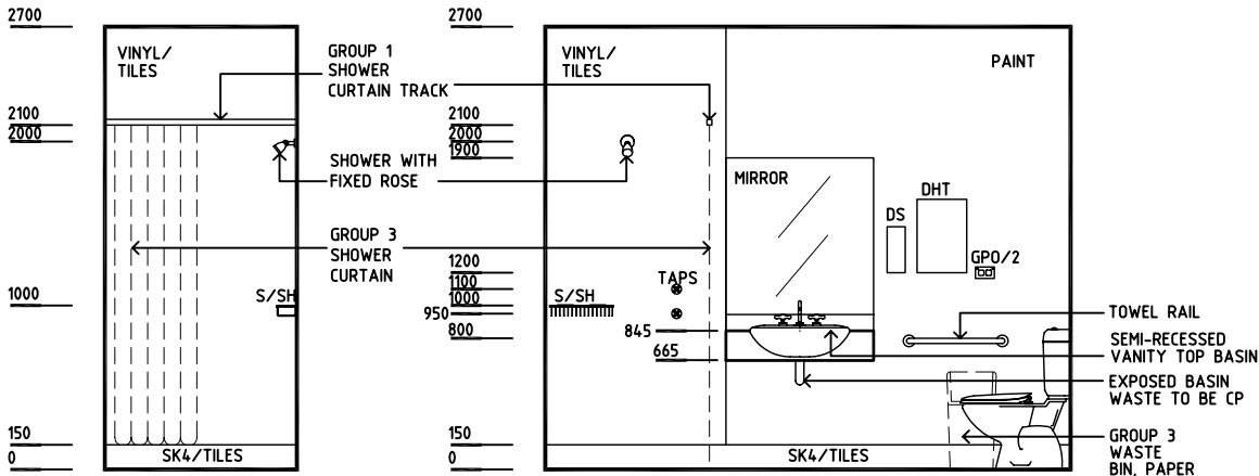
ELEVATION 3
