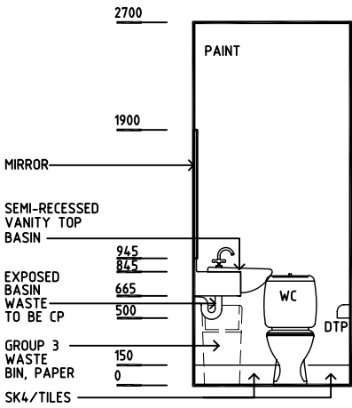
ELEVATION 1
