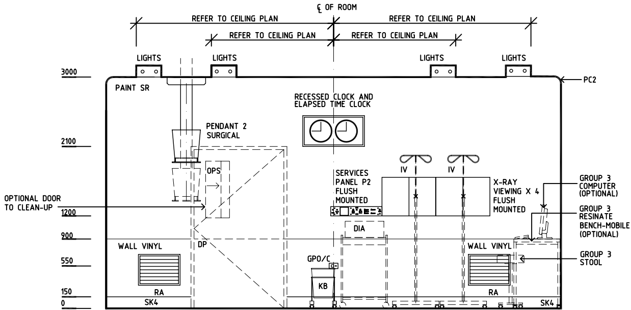
ELEVATION 4
