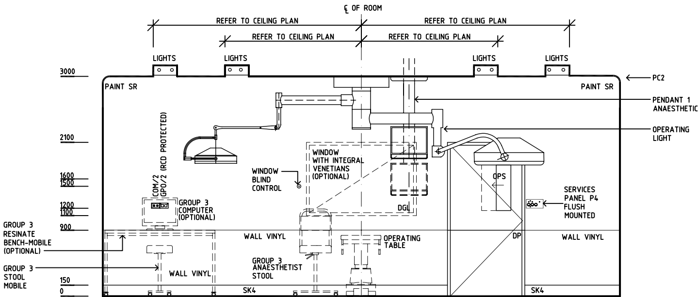
ELEVATION 1
