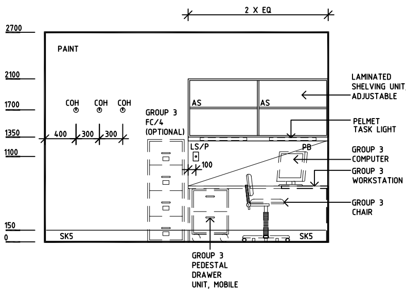
ELEVATION 4
