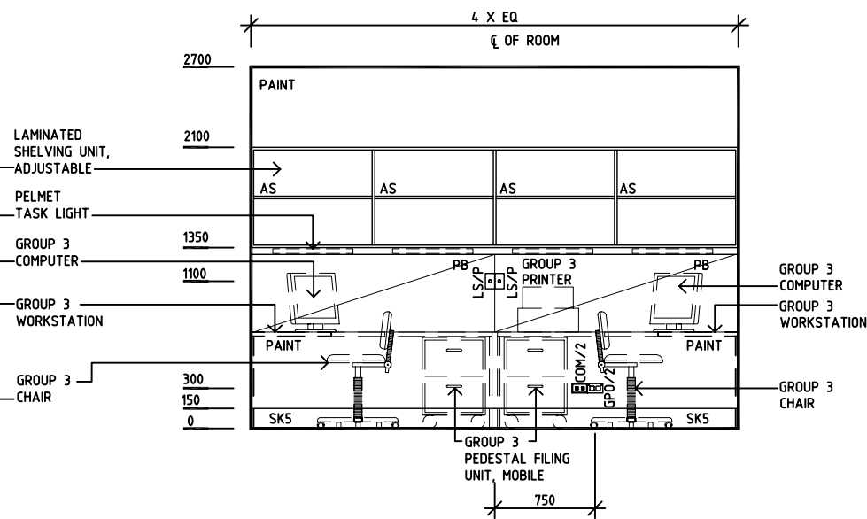
ELEVATION 2
