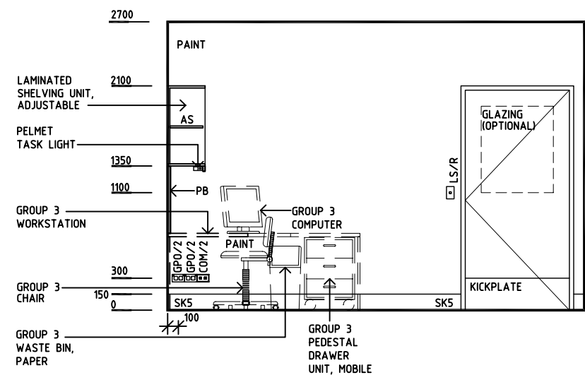
ELEVATION 3
