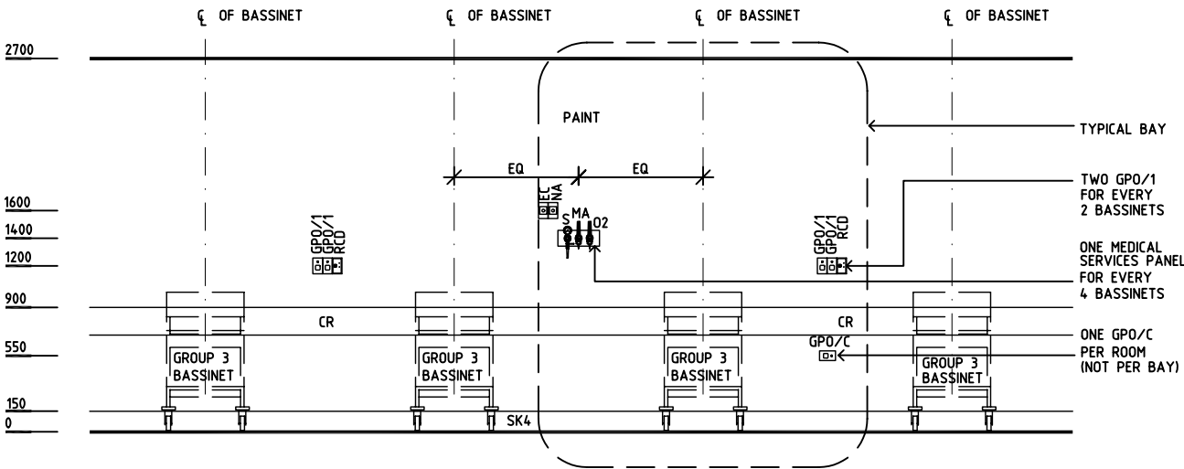
ELEVATION 1
