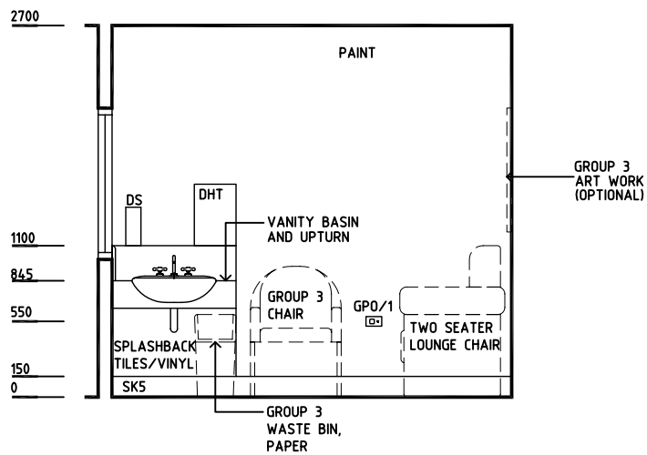
ELEVATION 3
