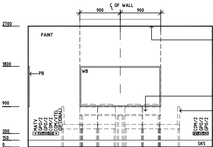
ELEVATION 1
