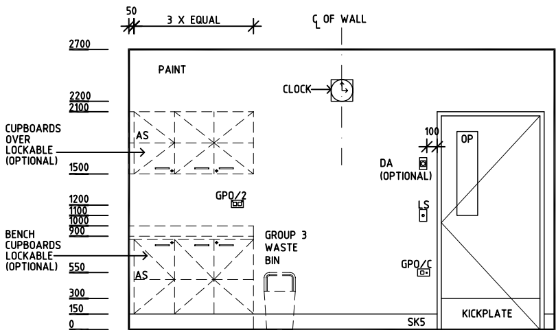
ELEVATION 3
