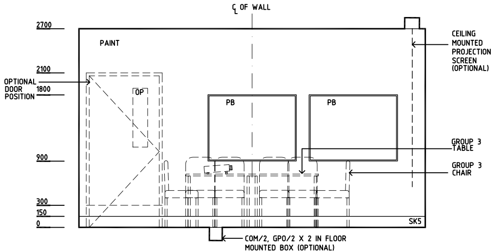
ELEVATION 4
