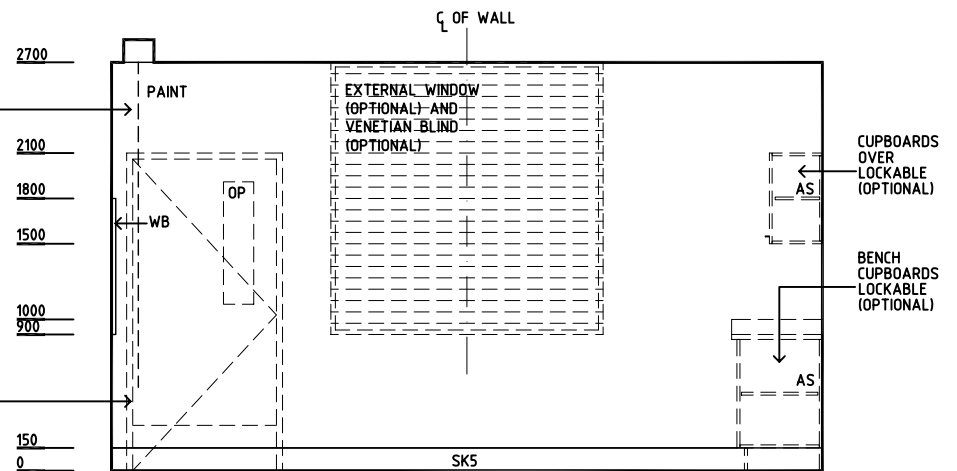
ELEVATION 2
