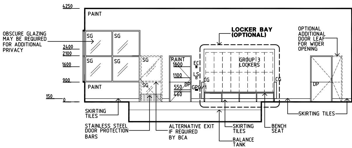
ELEVATION 1 1:100
