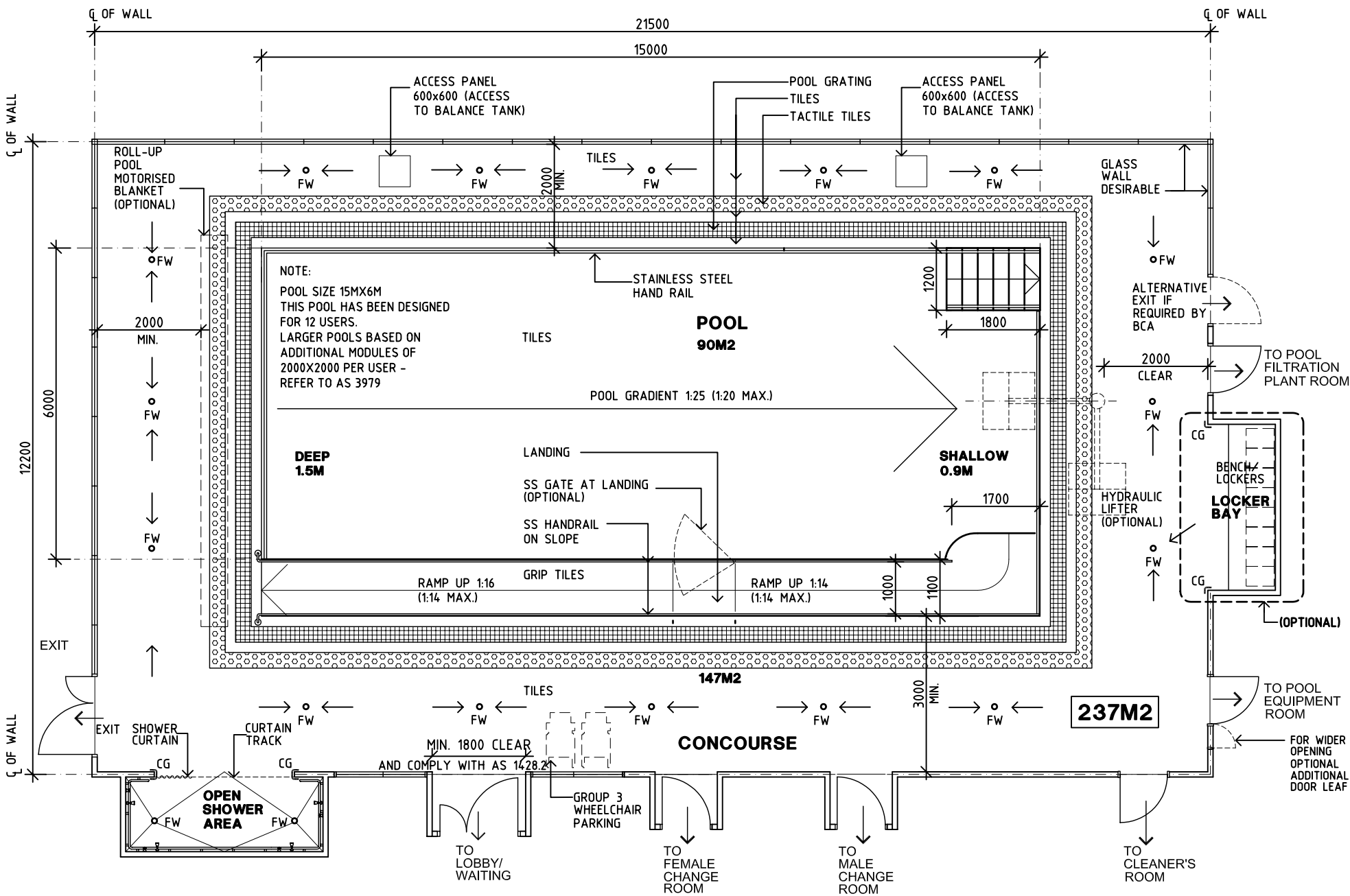
PLAN 1:100
