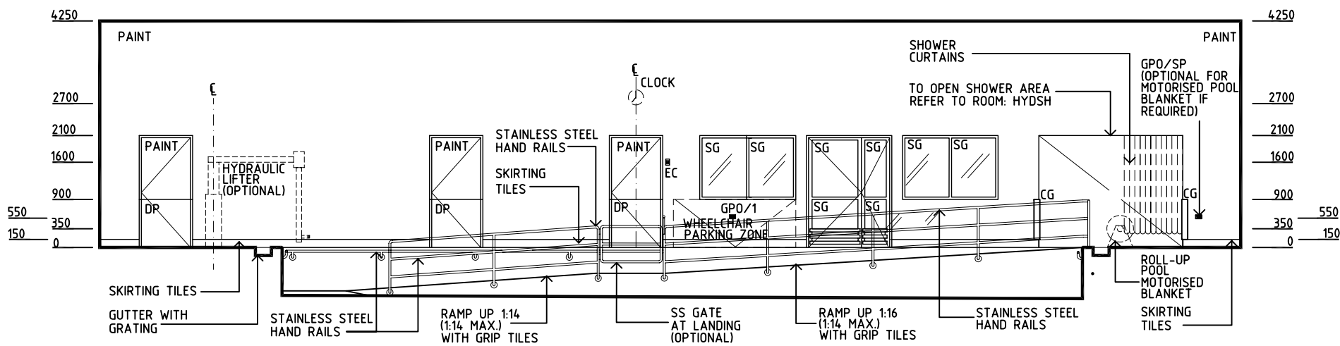
ELEVATION 2 1:100
