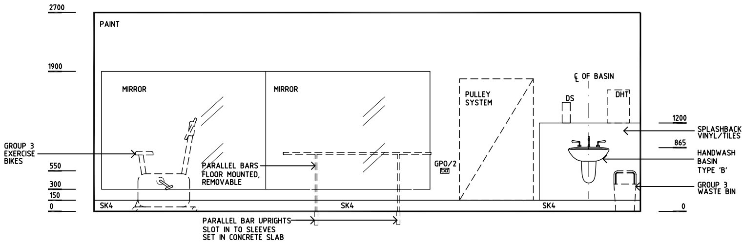
ELEVATION 2
