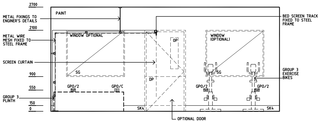
ELEVATION 1
