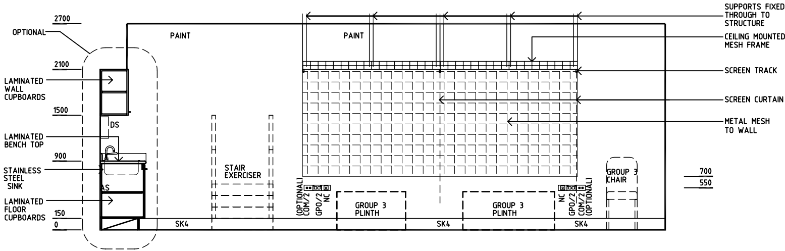
ELEVATION 4
