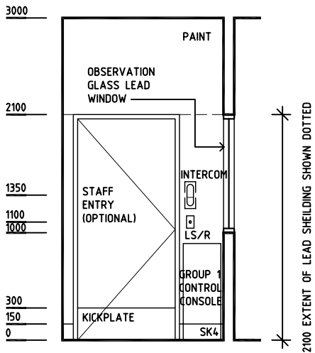
ELEVATION 6
