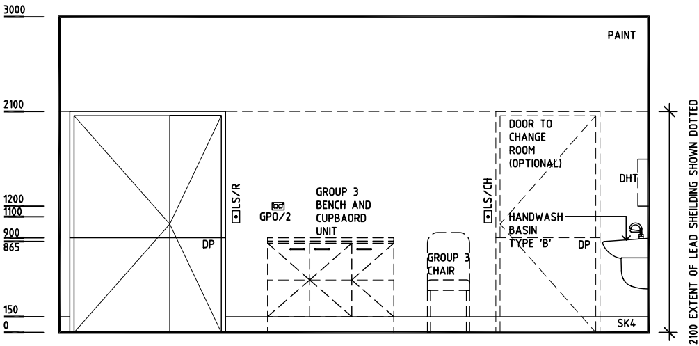
ELEVATION 3
