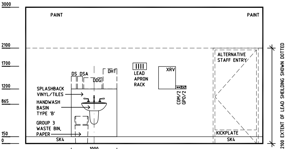
ELEVATION 4
