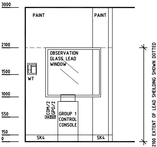
ELEVATION 5
