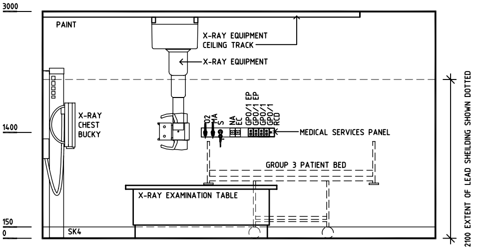
ELEVATION 2
