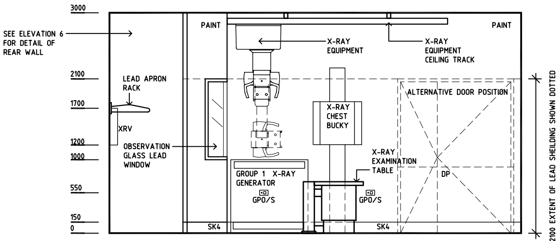
ELEVATION 1
