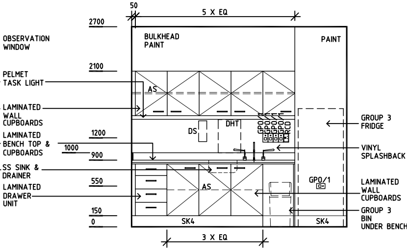
ELEVATION 4
