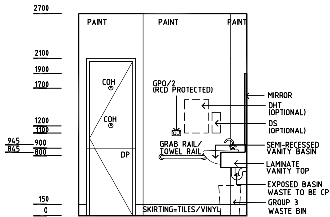
ELEVATION 4
