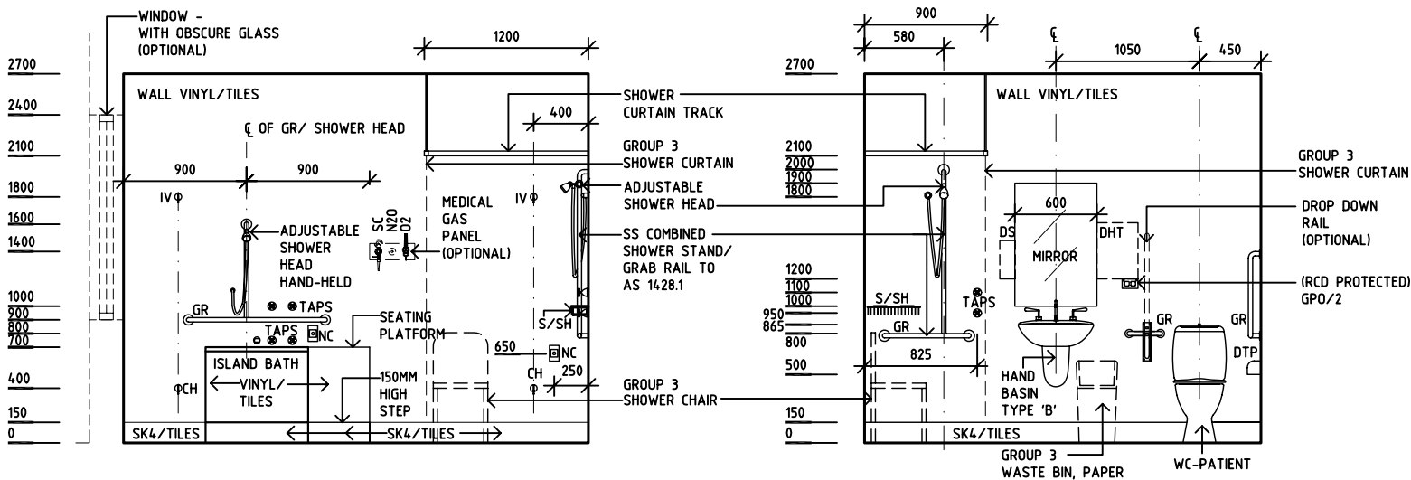
ELEVATION 3
