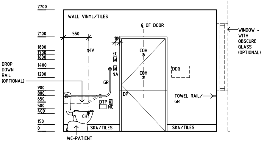
ELEVATION 1
