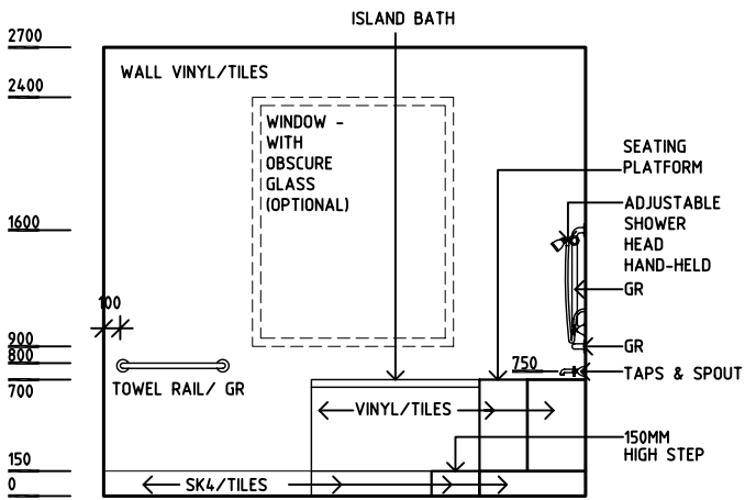
ELEVATION 2
