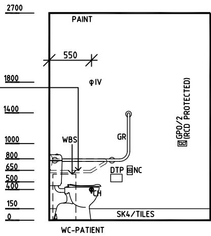
ELEVATION 4
