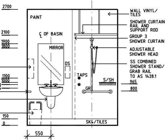
ELEVATION 2
