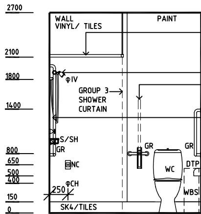
ELEVATION 3
