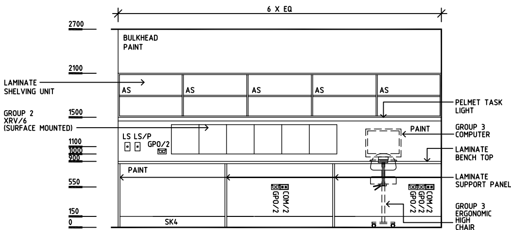
ELEVATION 3
