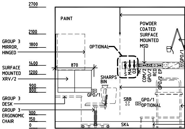
ELEVATION 1
