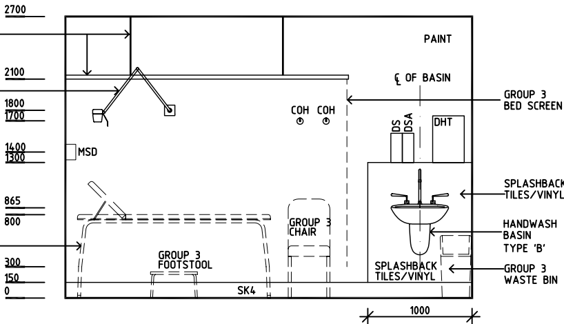
ELEVATION 2
