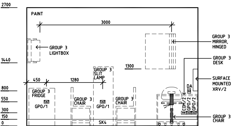
ELEVATION 4
