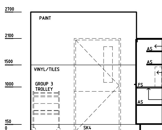
ELEVATION 1
