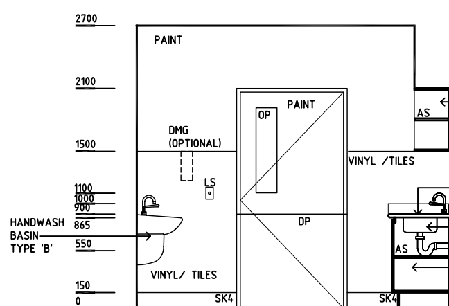
ELEVATION 1
