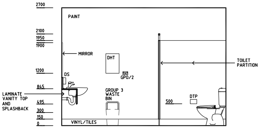
ELEVATION 3
