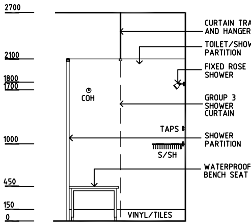
ELEVATION 6
