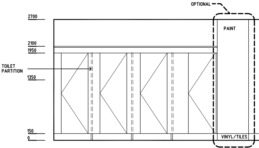
ELEVATION 7
