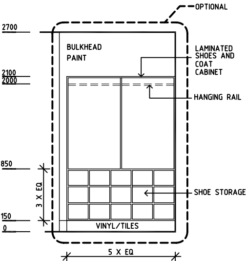
ELEVATION 5
