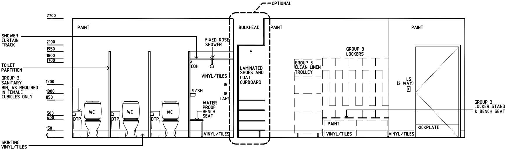
ELEVATION 4
