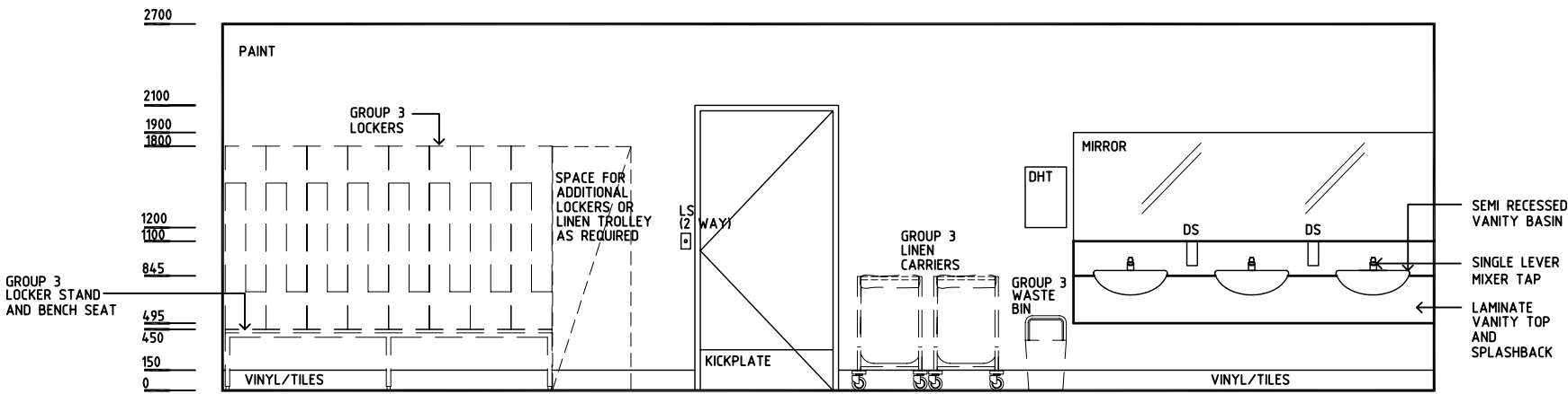
ELEVATION 2
