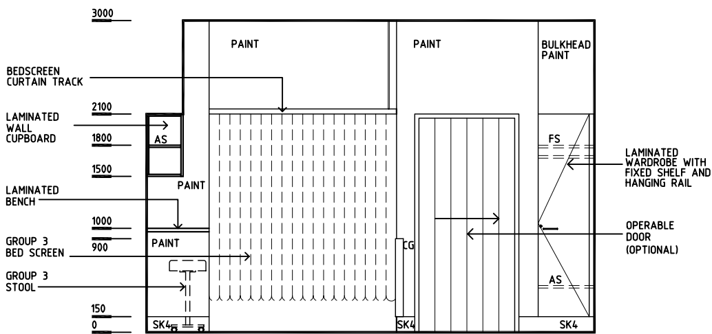
ELEVATION 4
