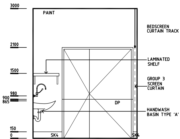
ELEVATION 5
