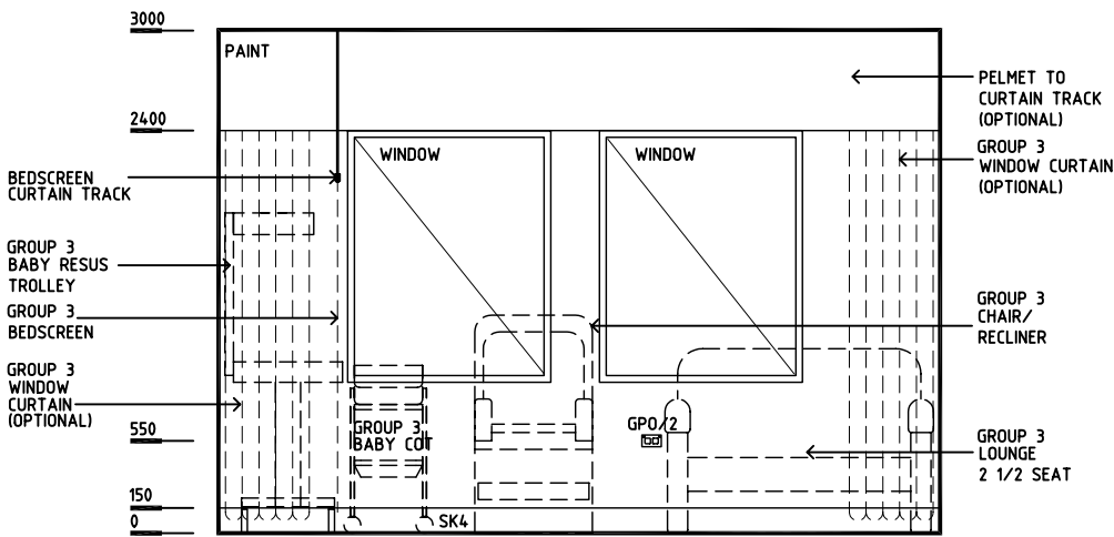
ELEVATION 2
