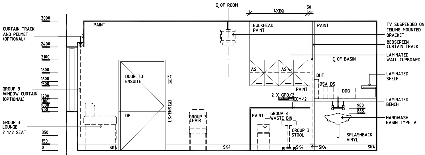
ELEVATION 3
