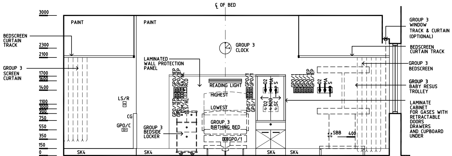
ELEVATION 1
