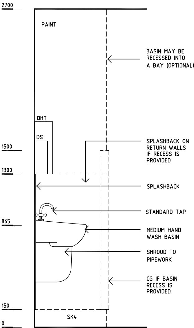
ELEVATION 2
