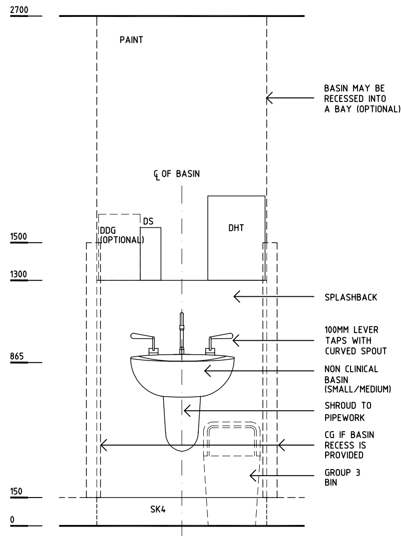
ELEVATION 1
