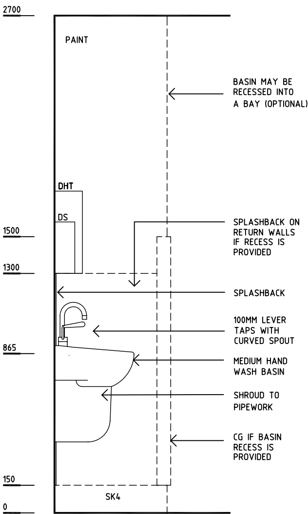
ELEVATION 2
