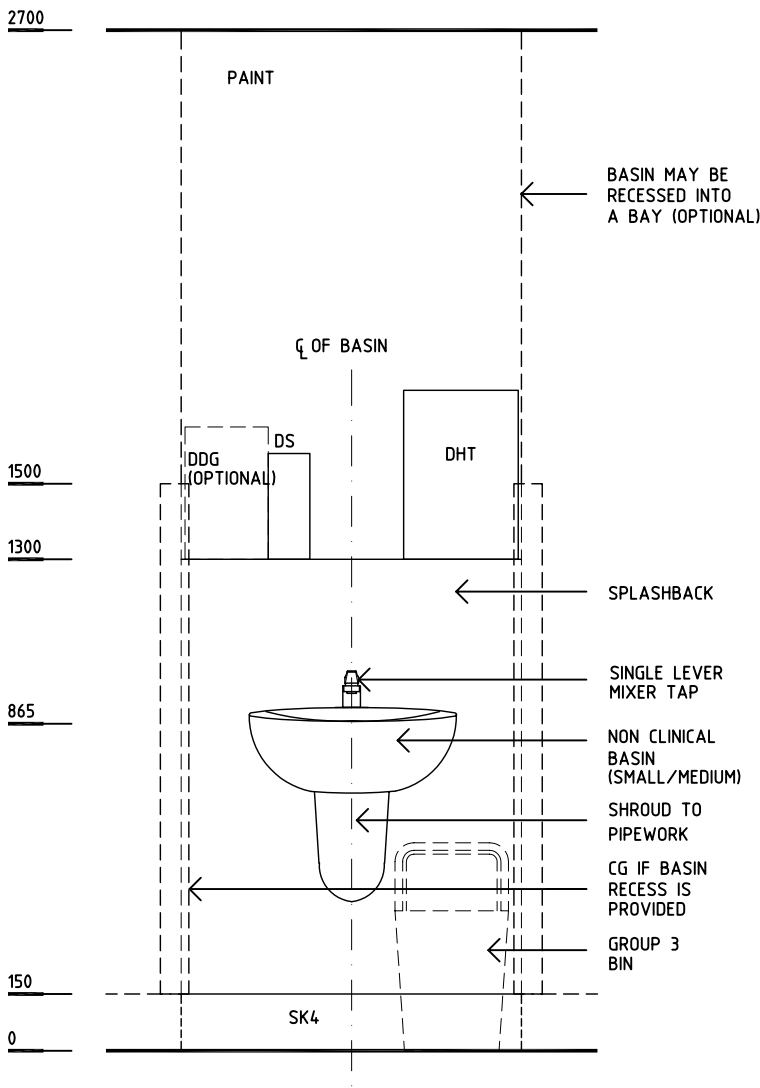
ELEVATION 1
