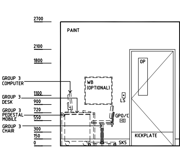
ELEVATION 3
