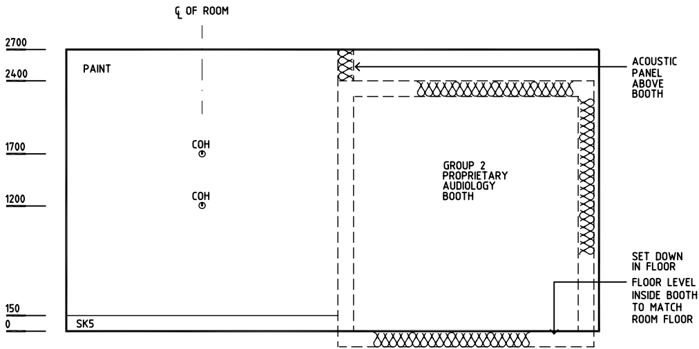
ELEVATION 4
