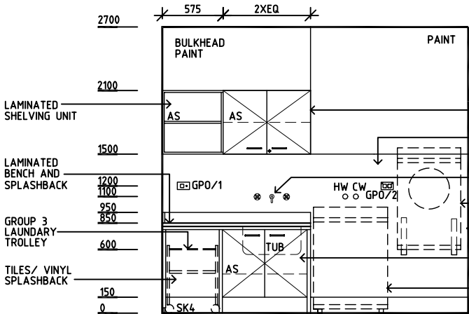
ELEVATION 1
