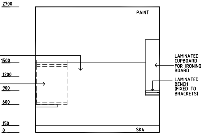
ELEVATION 2
