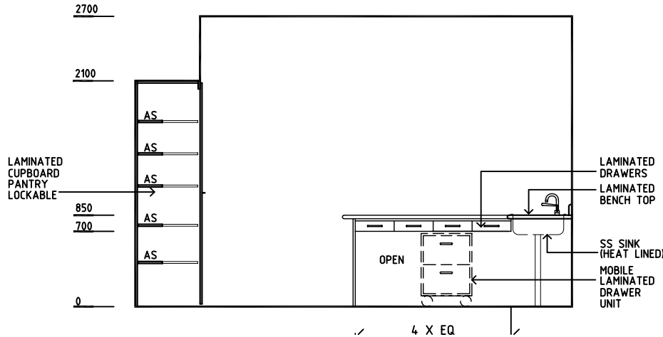
ELEVATION 4
